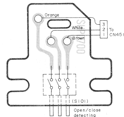
• Laser switch P.C.B.
